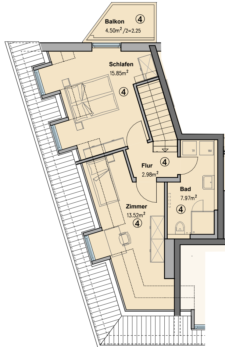
DG - Wohnung 4
