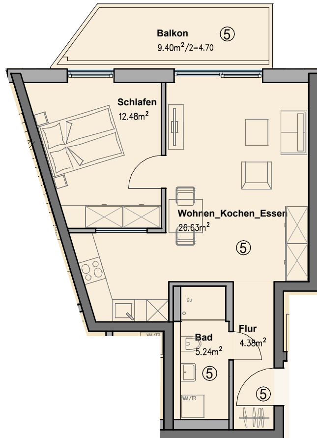
2.OG - Wohnung 5
